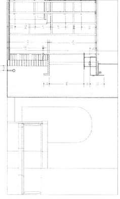
CORTE TRANSVERSAL
